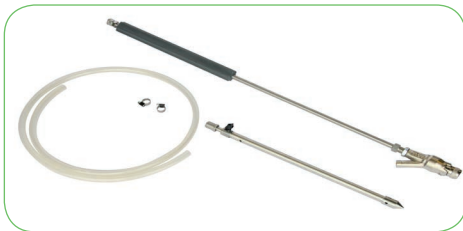
Gritstraallans van 900 mm met puntstraal-sproeier, snelkoppeling en aanzuigbuis geschikt voor werkdruk \leq 350 bar en \leq 500 bar code: 1.258.225.00xxx code: 1.258.225.15xxx
