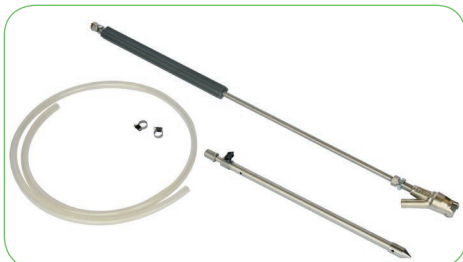
Gritstraallans van 900 mm met vlakstraal-sproeier, snelkoppeling en aanzuigbuis geschikt voor werkdruk \leq 350 bar en \leq 500 bar code: 1.258.229.00xxx code: 1.258.229.15xxx
